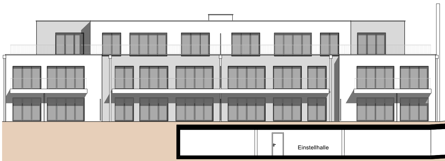
WESTFASSADE
