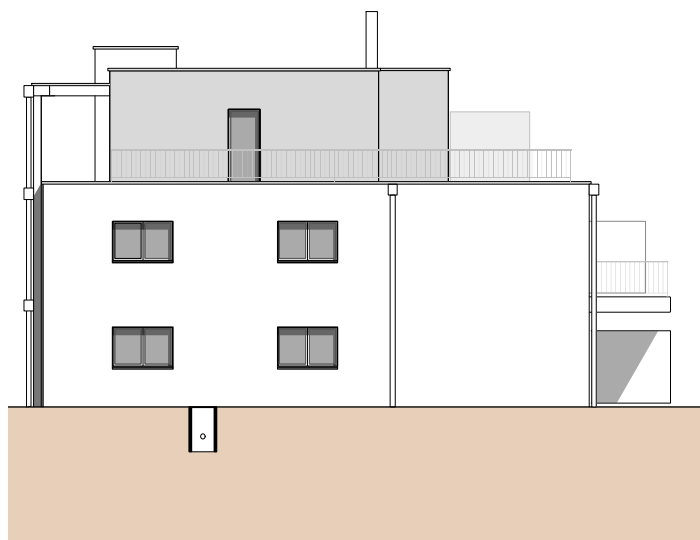
NORDFASSADE
