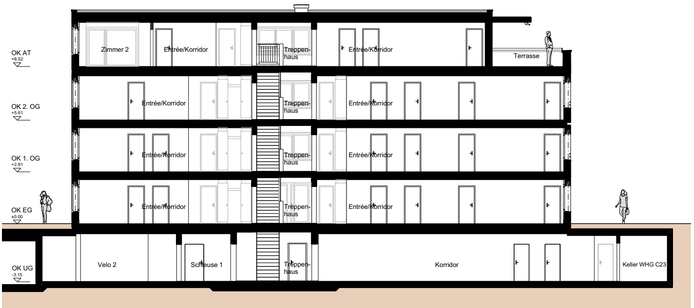
Schnitt A-A
