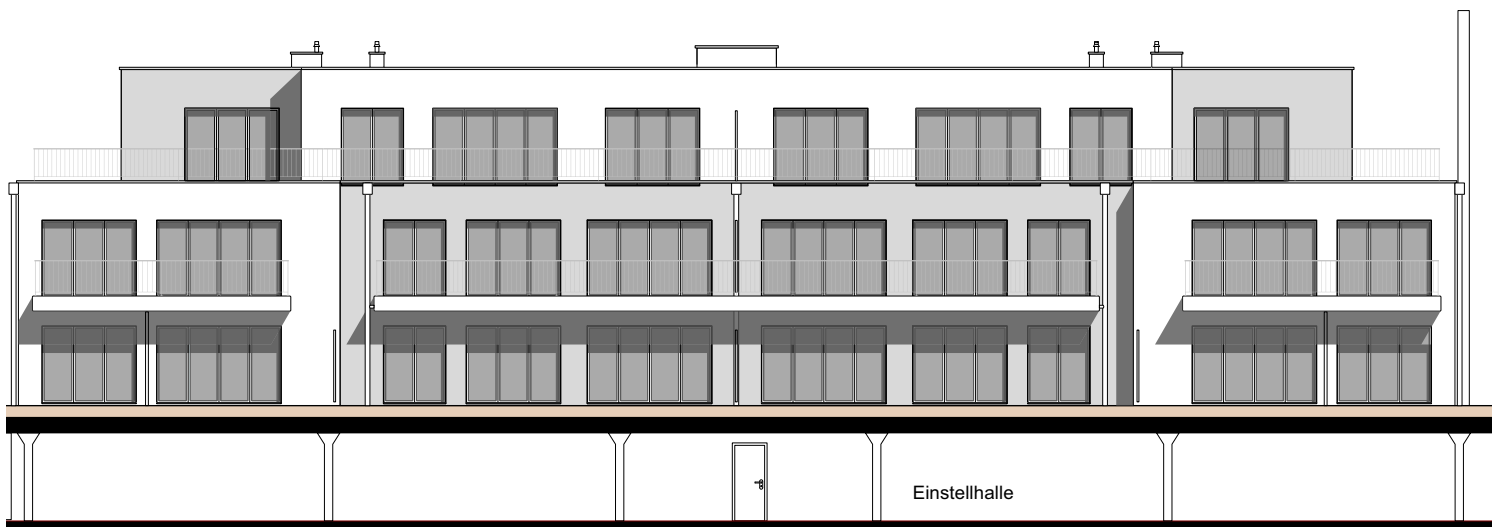
WESTFASSADE
