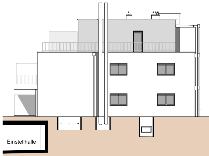
SÜDFASSADE
