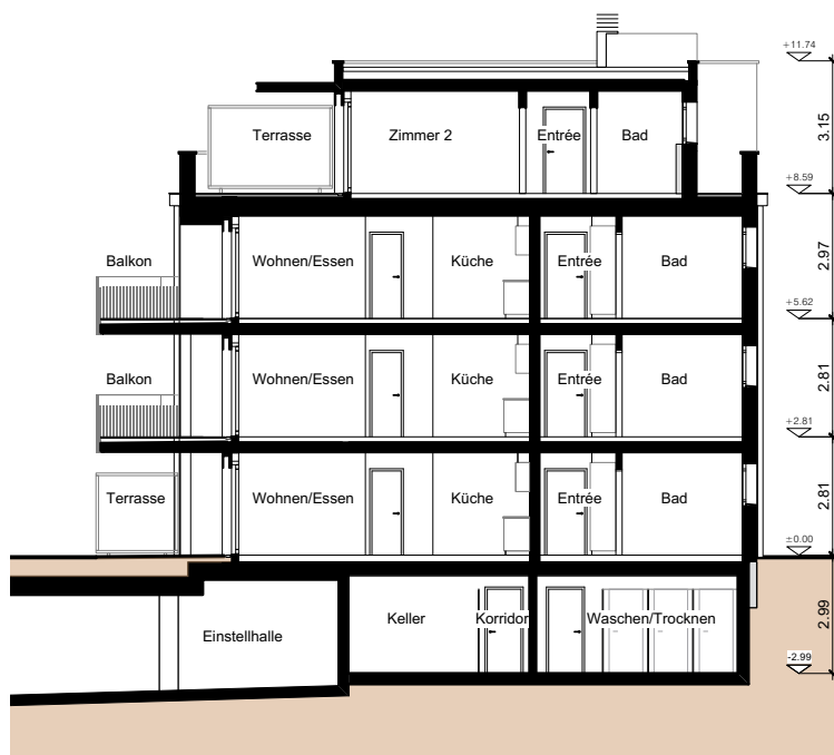
SCHNITT 2-2
