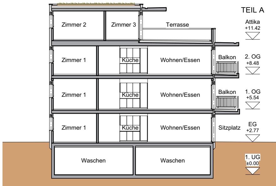
Querschnitt B-B
