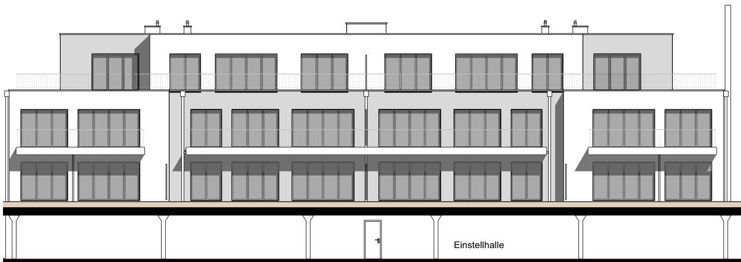
WESTFASSADE
