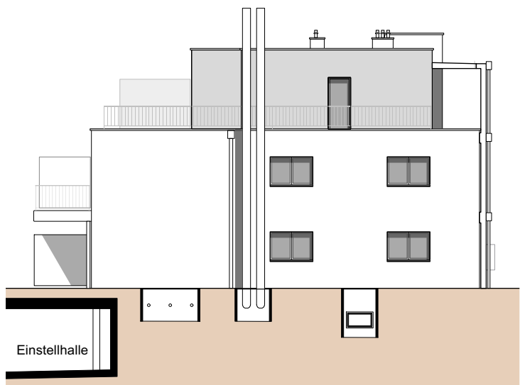
SÜDFASSADE
