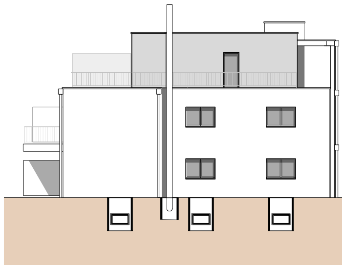
SÜDFASSADE
